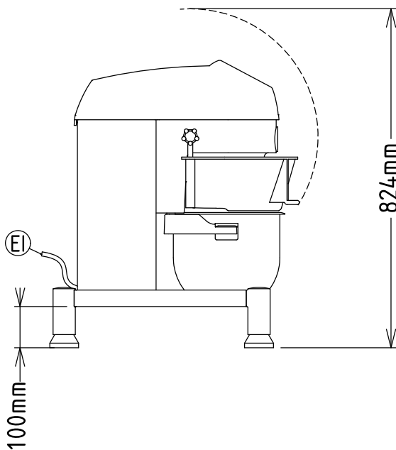
Zij aanzicht
